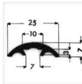
Bordures avec raccord vissé
